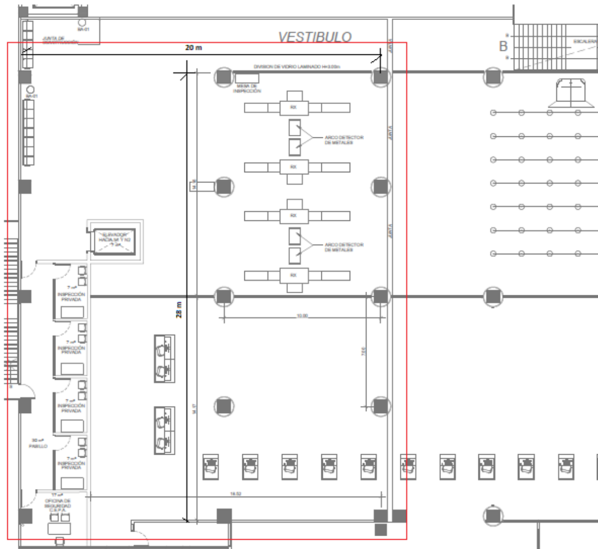
Ilustración 1 Ilustración 1 Plano del área de punto de inspección 5 e inmigración del edificio de la ampliación del AIES-SOARG. (28 x 20 metros aproximados)
