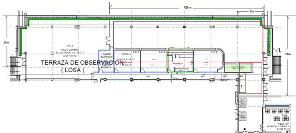
Ilustración 1 Plano del área de plaza de la comida para distribución de ductería (40 x 14 metros aproximados)
